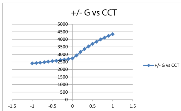
Comportamiento +/- G en 2700K
